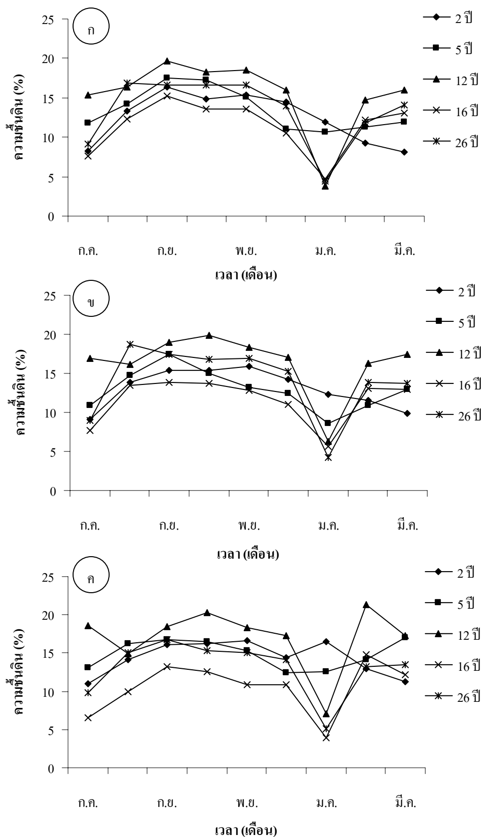
รูปผนวกที่ 3 เปรี่อ์เซ็นต์ความชื้นในดินที่ระดับความลึก 0-20 ซม. (ก) 20-40 ซม. (ข) และ 40-60 ซม. (ค) ในแปลงทดลองของต้นยางพาราในแต่ละช่วงอายุ
